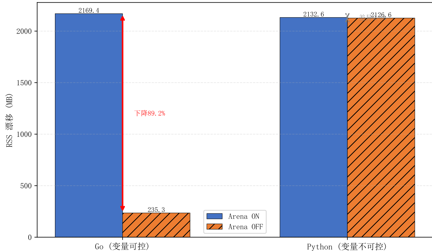
图 4-补充(b) 跨语言负对照验证: Arena 开关对 RSS 漂移的影响
