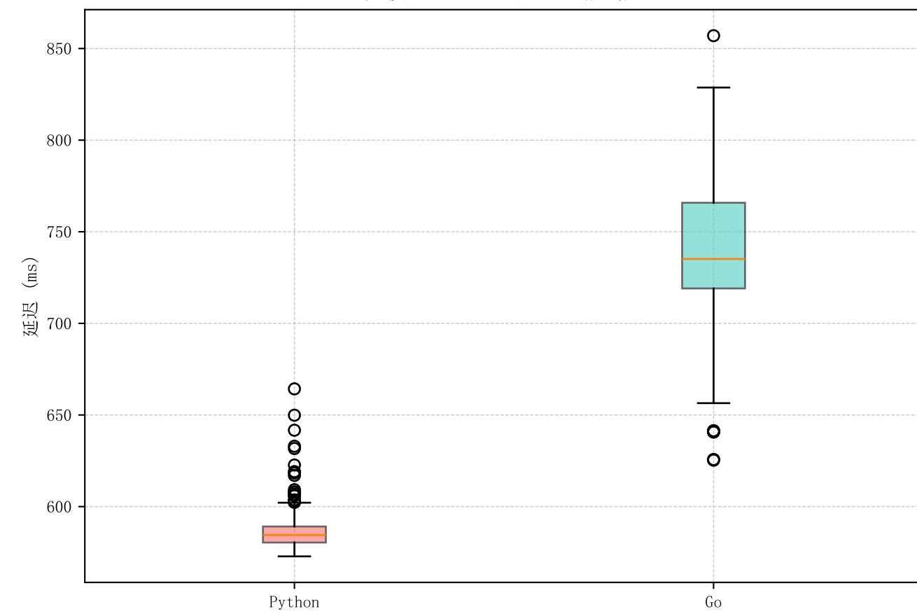
大模型 (YOLO11x) 延迟箱线图
