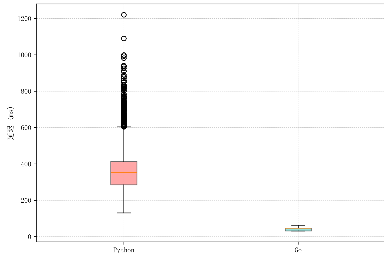
轻模型 (YOLO11n) 延迟箱线图
