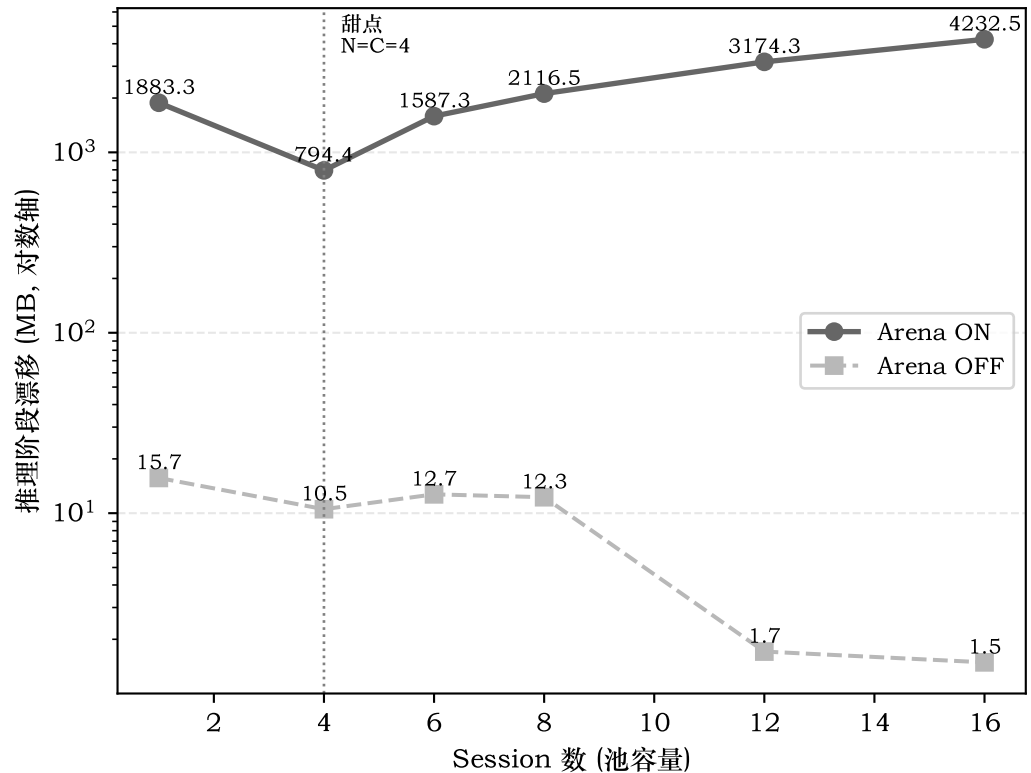
(b) 甜点效应 (并发Run()=4)
