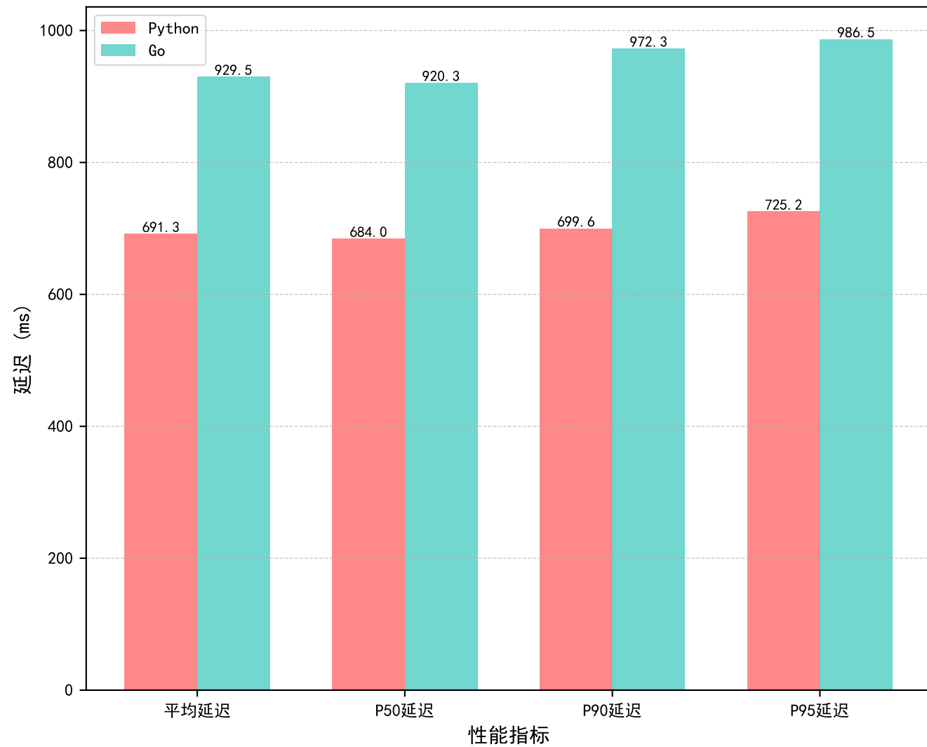
大模型（YOLO11x）性能对比
