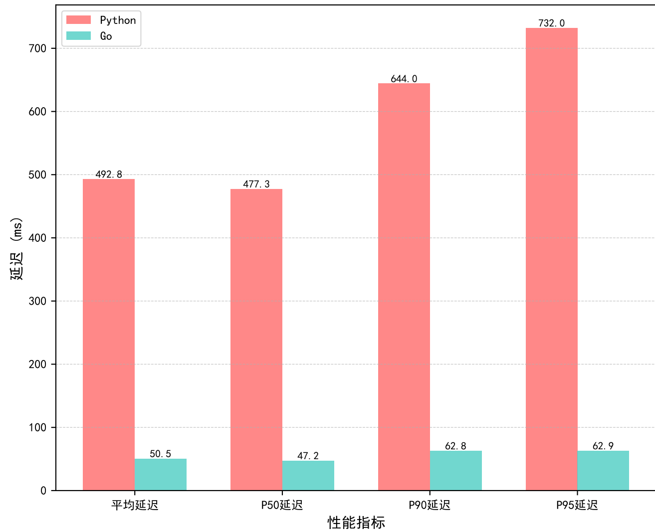
轻模型（YOLO11n）性能对比
