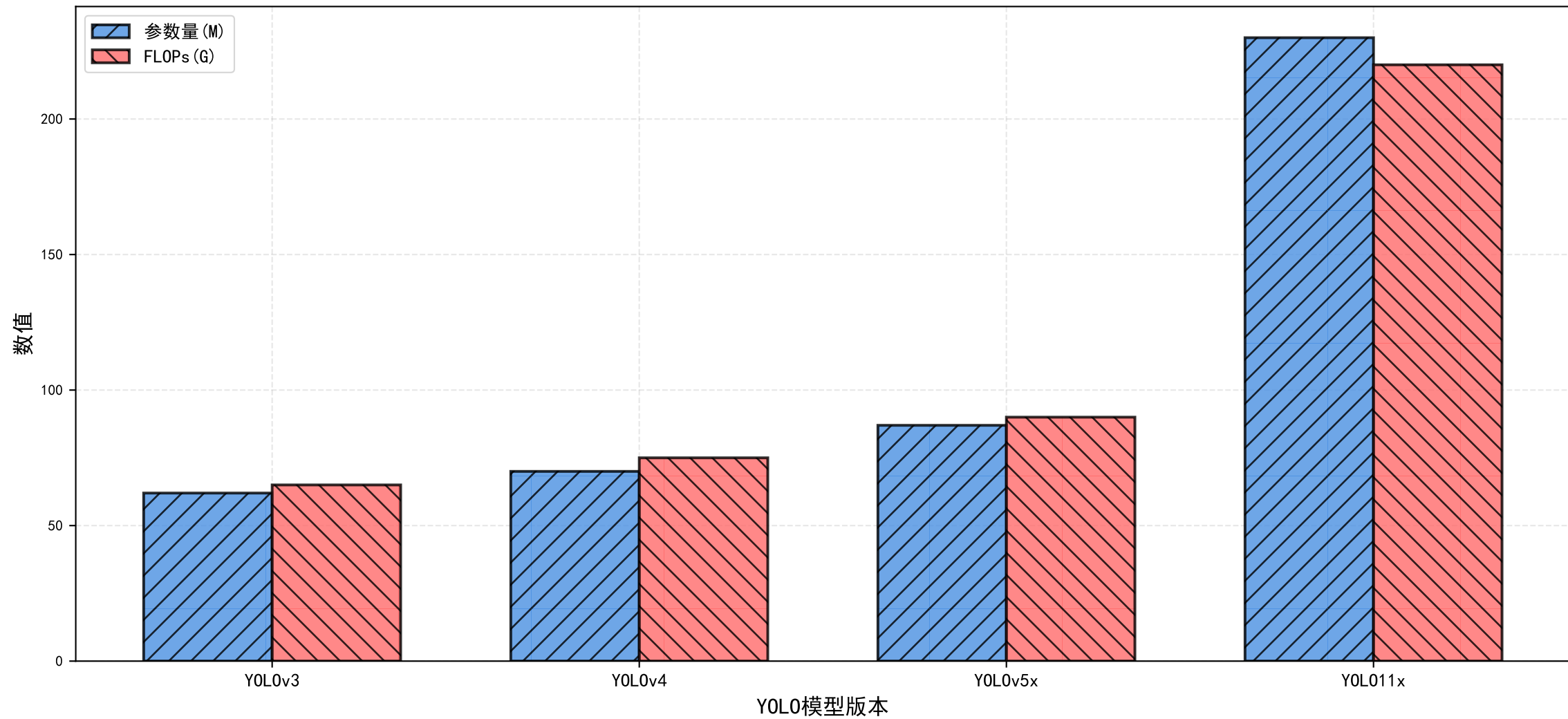
YOLO系列模型参数量与FLOPs演化趋势
