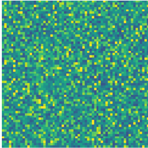
pure noise
