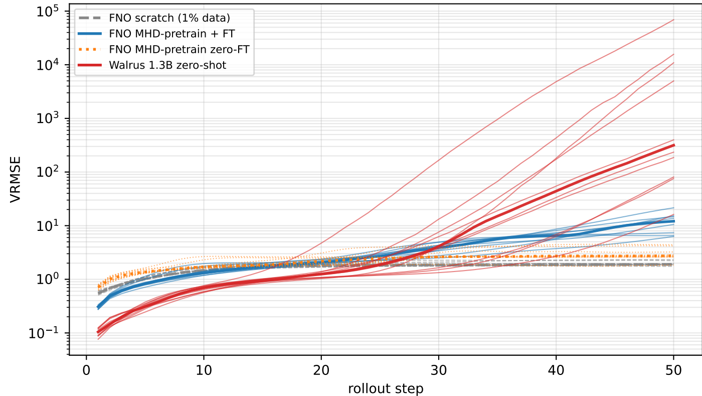
Per-trajectory rollout VRMSE: all 10 trajectories per method
