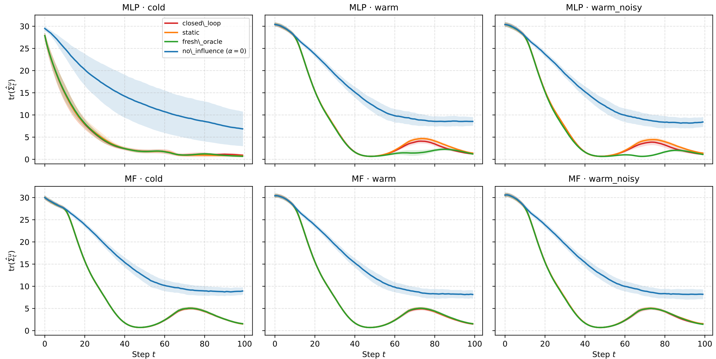
H7: \text{tr}(\hat{\Sigma}) при разных моделях и инициализациях (N=300, T=100, seeds=30)
