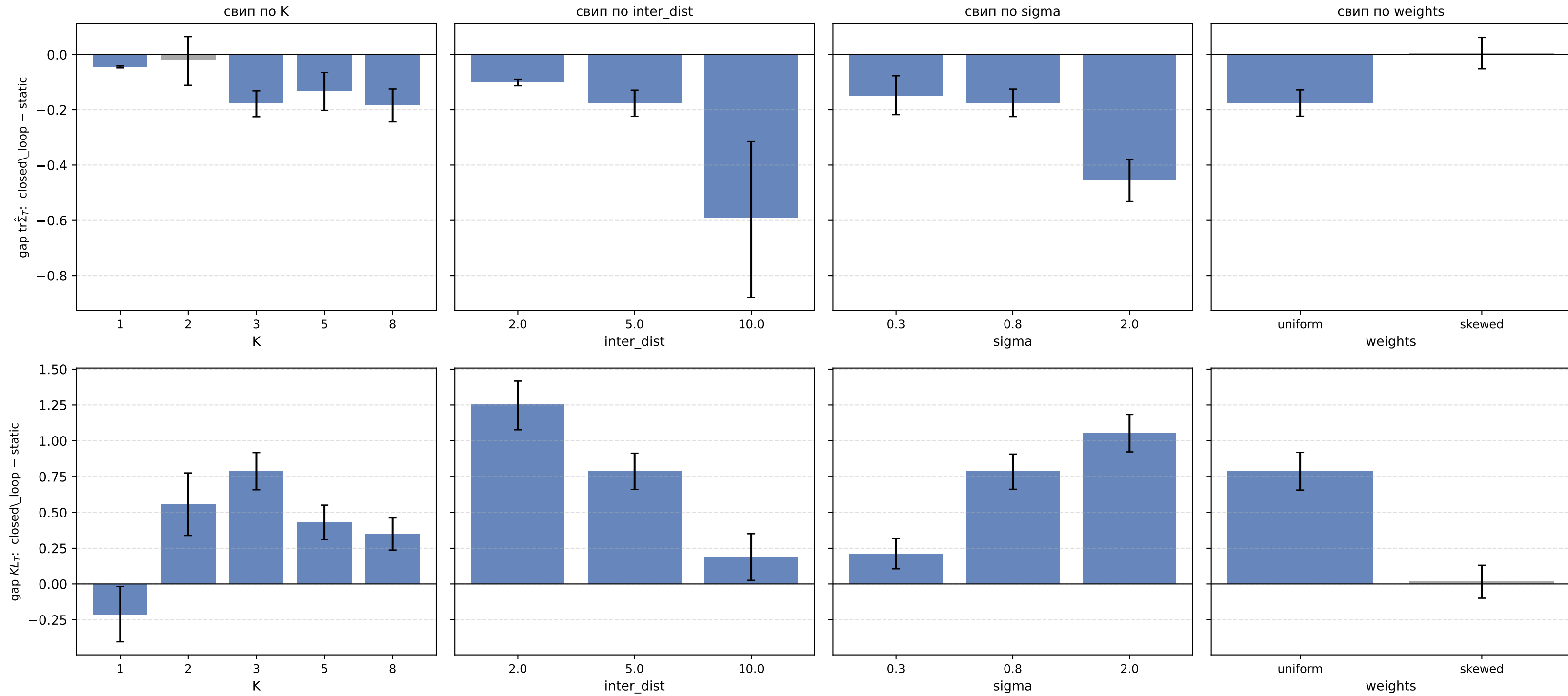
Н8.В: разрыв (closed\_loop – static) по 4 осям начального распределения (MLP-warm, синий — 95% CI исключает 0)
