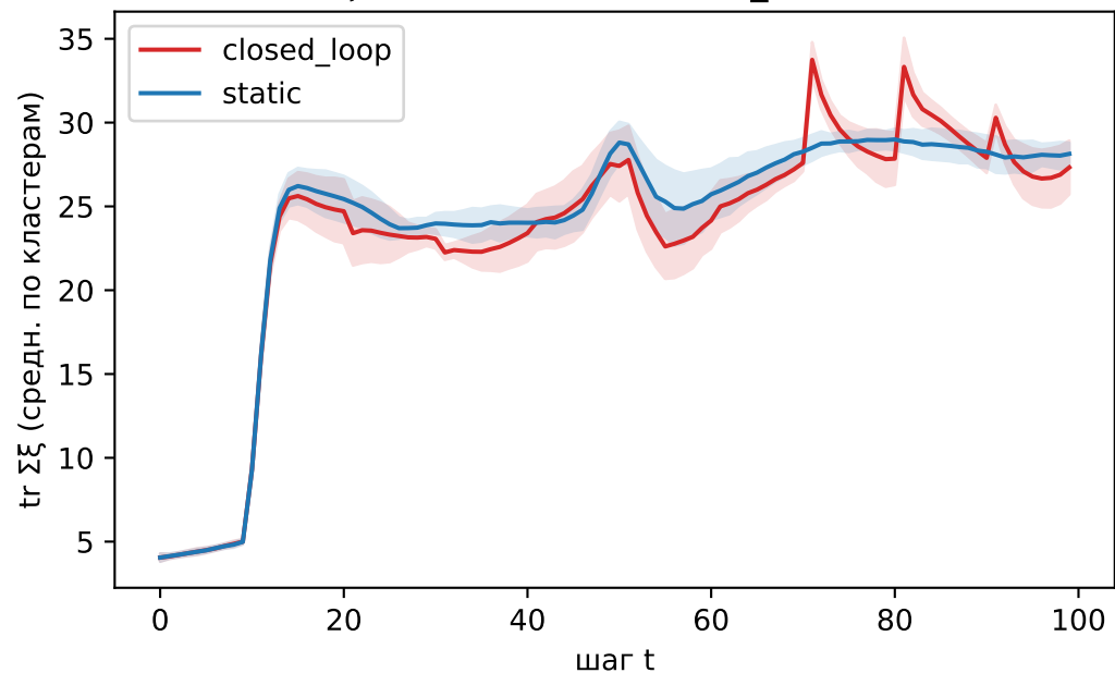
tr \Sigma\xi (показанное) — seen_filter=True
