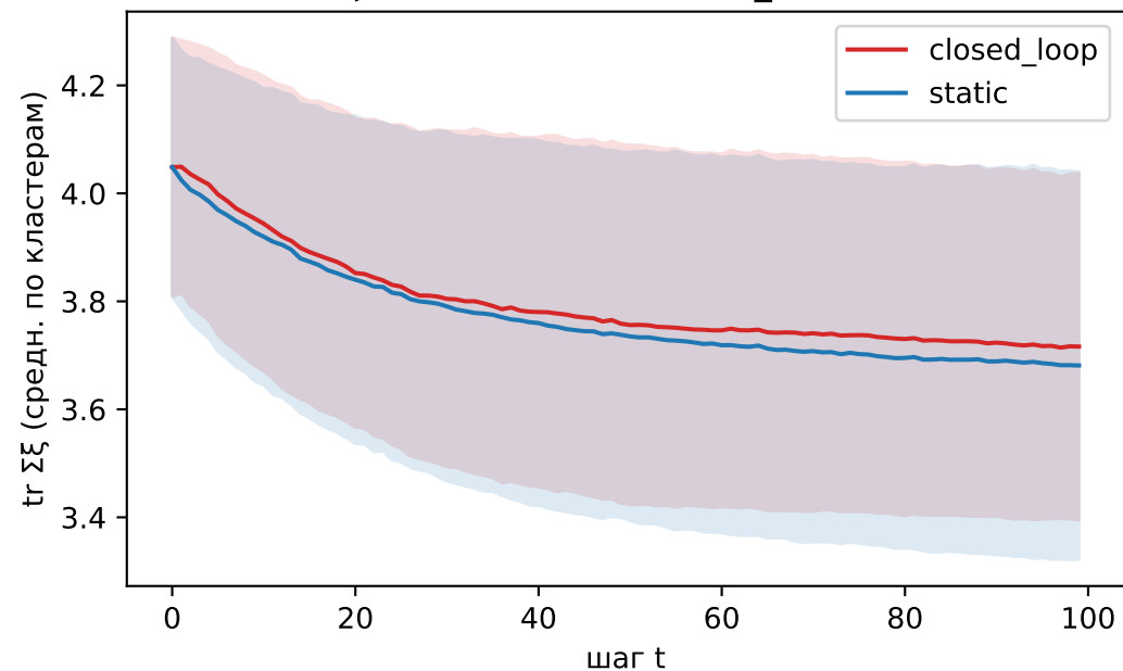
tr \Sigma\xi (показанное) — seen_filter=False
