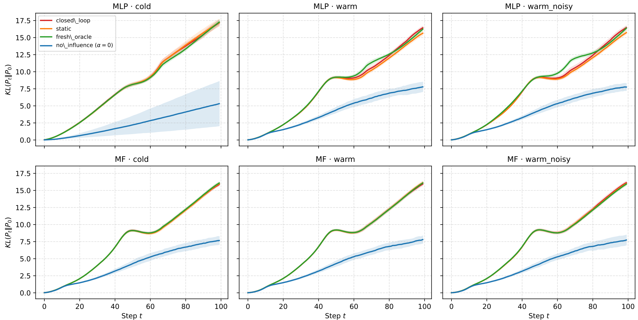
H7: KL-дивергенция при разных моделях и инициализациях (N=300, T=100, seeds=30)
