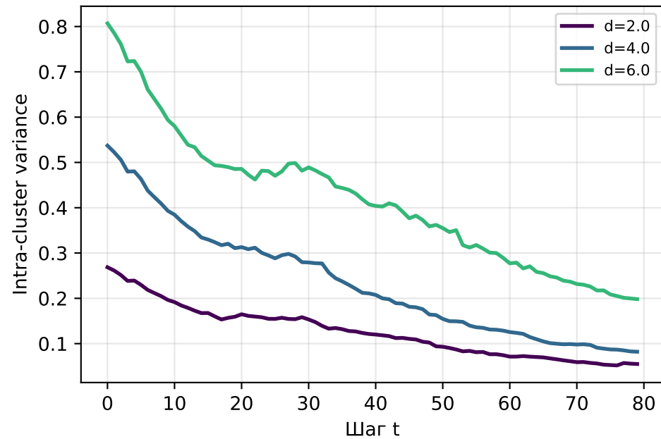
К=4 компонент
