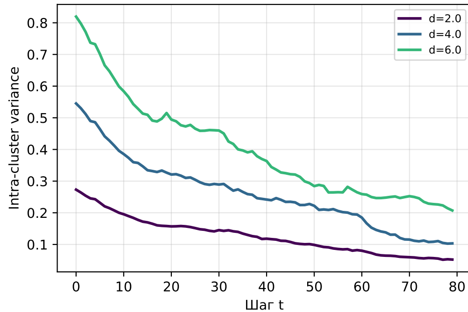
К=2 компонент
