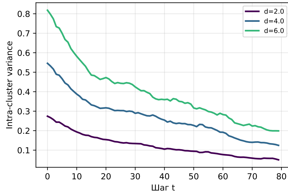
К=1 компонент
