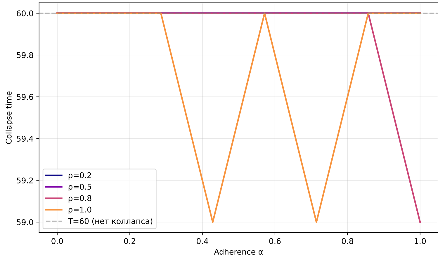
H4: Collapse time как функция \alpha
