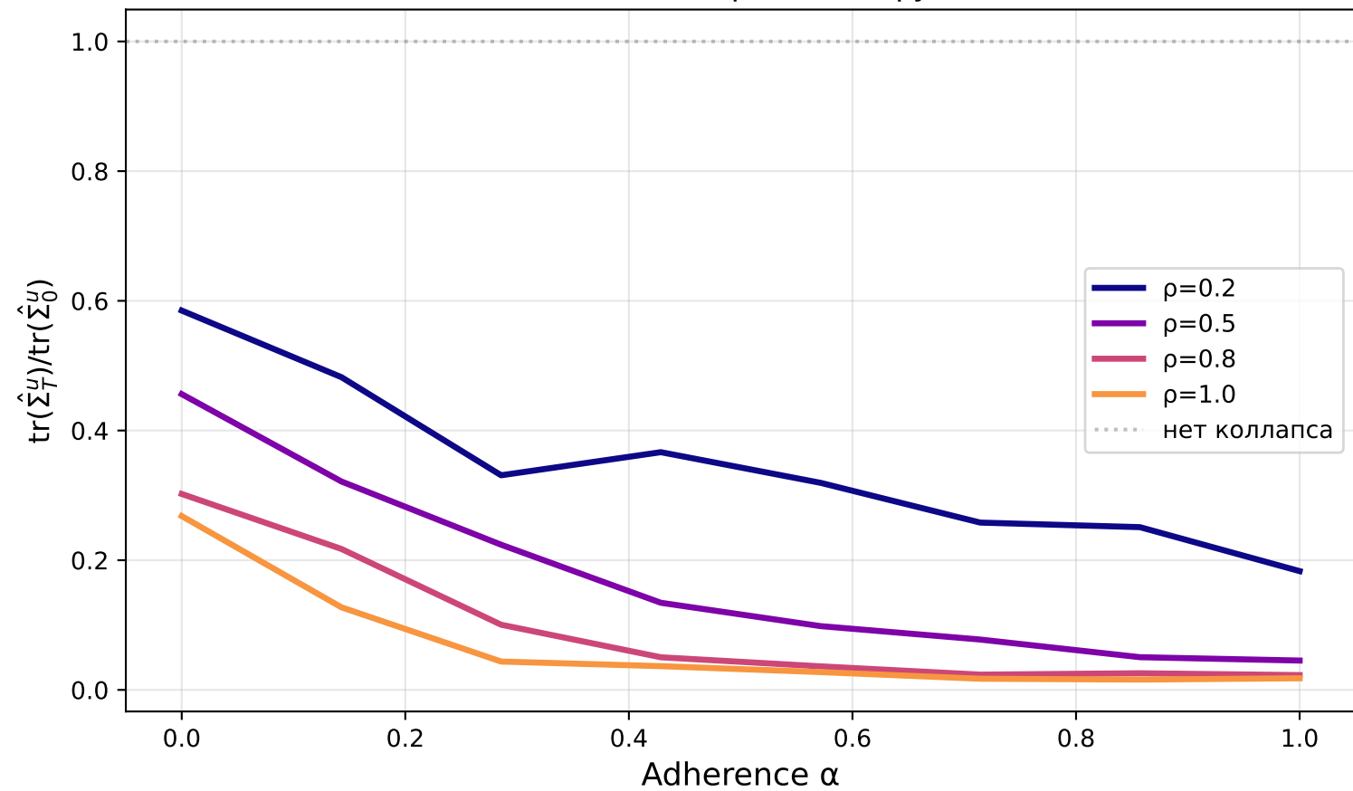
Н4: Коллапс дисперсии как функция \alpha
