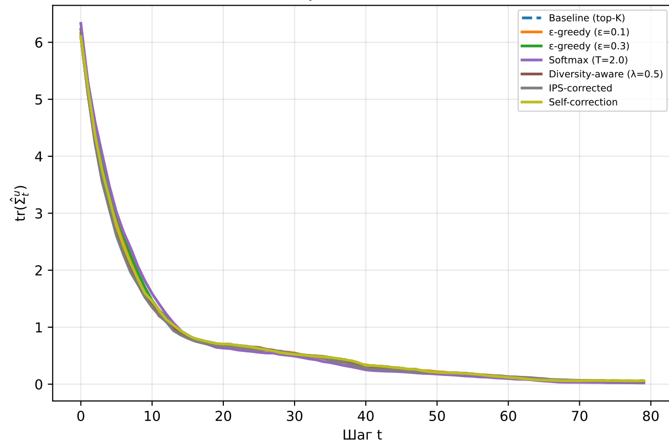
H5: \text{tr}(\hat{\Sigma}_t^u) по интервенциям
