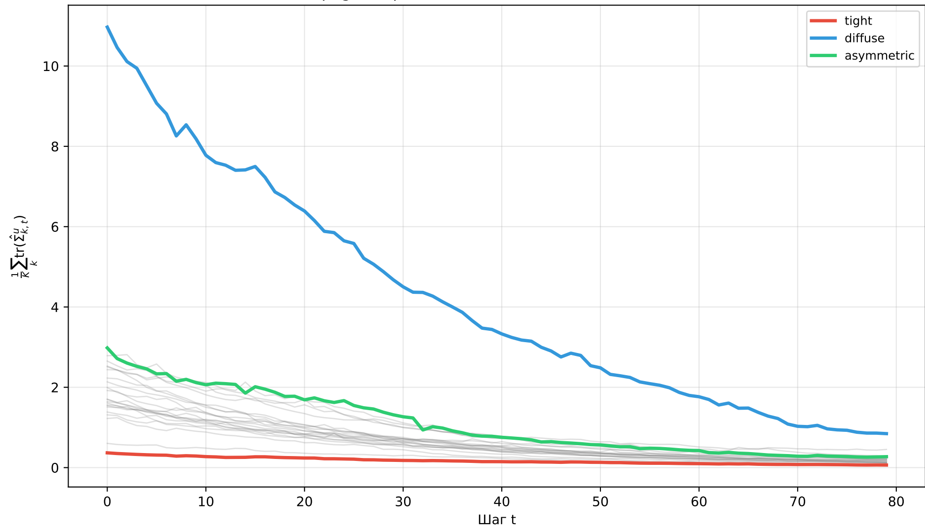
T.2: Spaghetti plot — 23 инициализаций сходятся к 0
