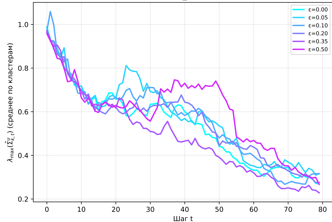
T.5b: Траектории \lambda_{\max} при разных \varepsilon
