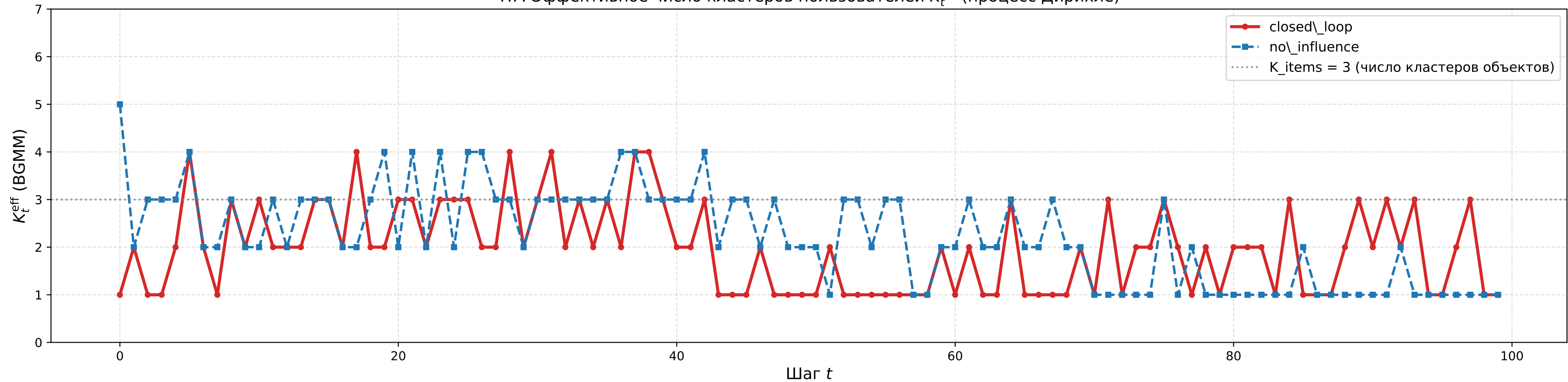
Т.7: Эффективное число кластеров пользователей K_t^{\text{eff}} (процесс Дирихле)
