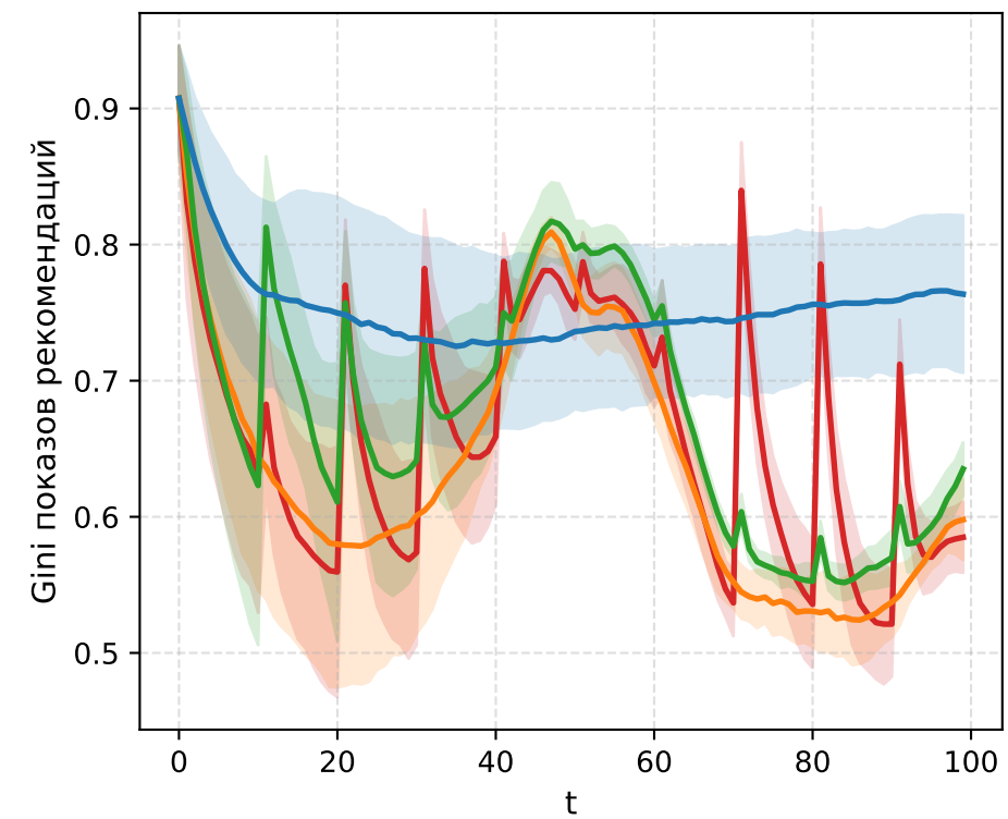
Н1+Н3 диагностика: 6 метрик во всех четырёх режимах (N=300, T=100, 8 seeds, \alpha=0.7 , \beta=0.005 )
