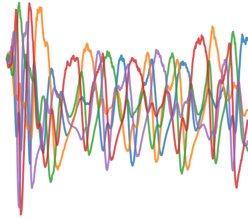
Lorenz96 (5D)
