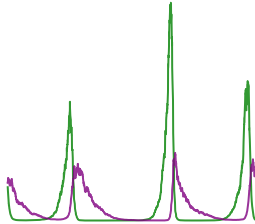
Lotka-Volterra
