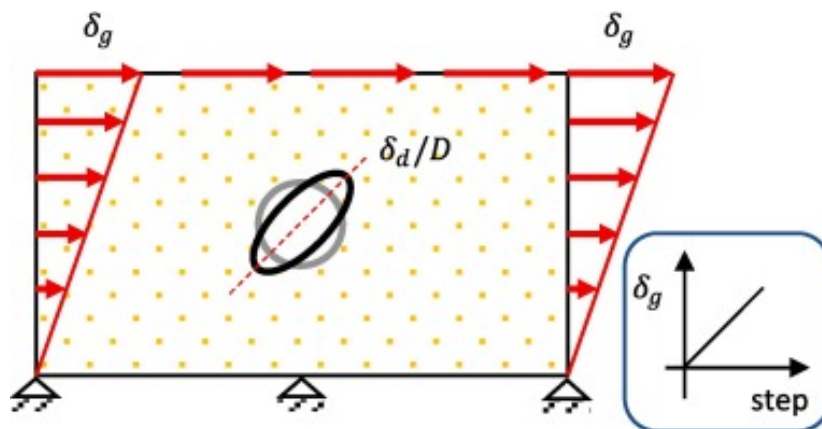
Σχήμα 3.10: Αριθμητικό Προσομοίωμα Ανάλυσης Pushover (Tsinidis κ.ά. 2024a)
