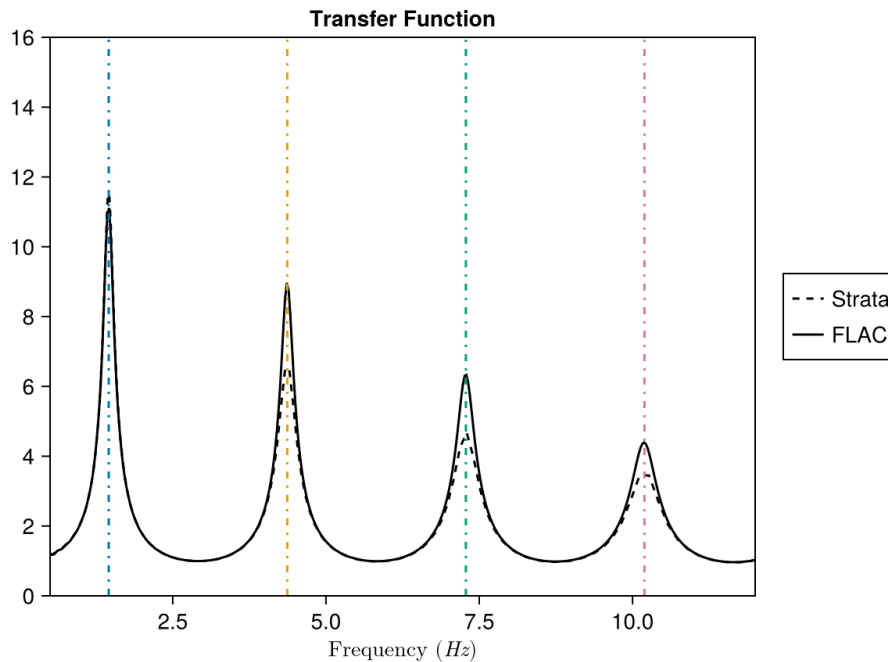
Σχήμα 3.5: Συνάρτηση Μεταφοράς Ελαστικής Ανάλυσης
