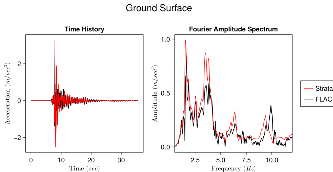
Σχήμα 3.8: Επιφανειακή Απόκριση Ελαστικής Στρωματοποιημένου Προσομοιώματος
