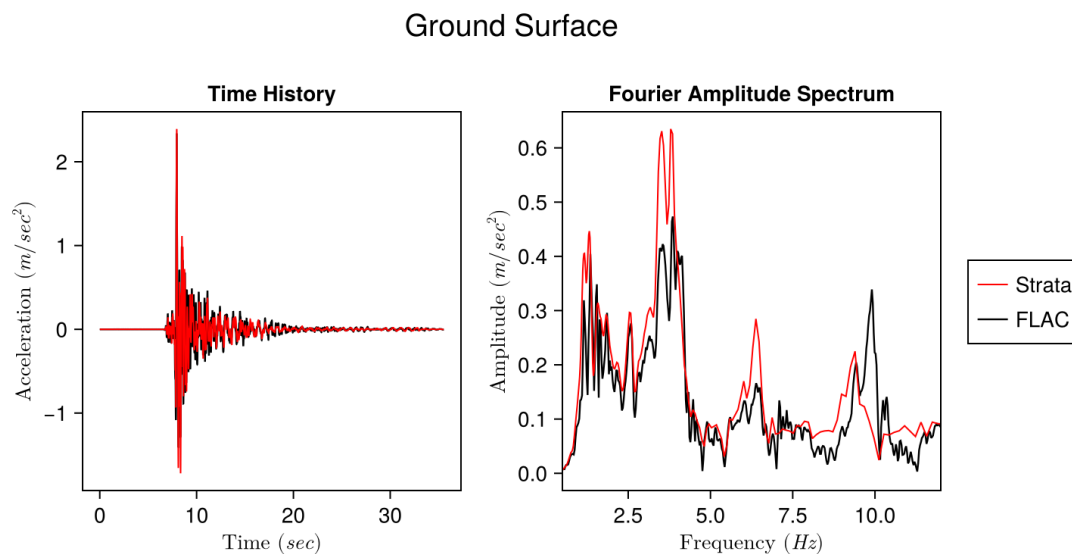
Σχήμα 3.6: Επιφανειακή Απόκριση Μη-Γραμμικής Ανάλυσης
