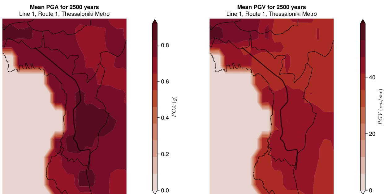
Σχήμα 2.16: Χάρτες Μέσων PGA-PGV Γεωλογίας-Κλίσης ESRM20
