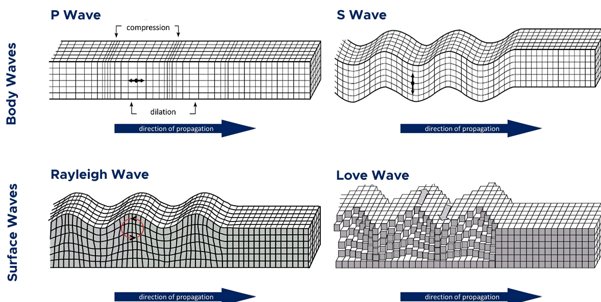
Σχήμα 2.1: Τύποι Σεισμικών Κυμάτων (Πηγή: LukeTriton κ.α. )
