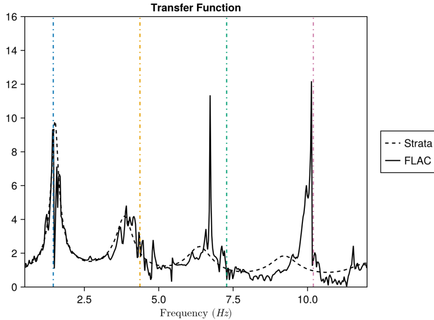
Σχήμα 3.9: Συνάρτηση Μεταφοράς Στρωματοποιημένου Προσομοιώματος
