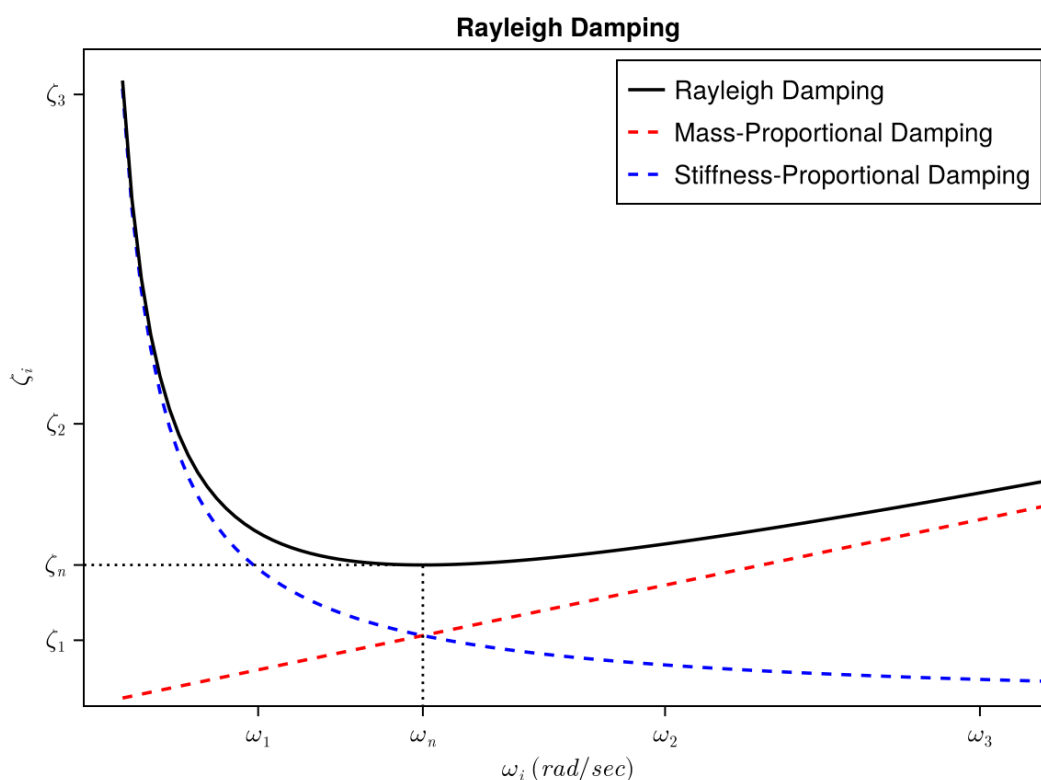
Σχήμα 3.1: Μητρική Απόσβεση Rayleigh
