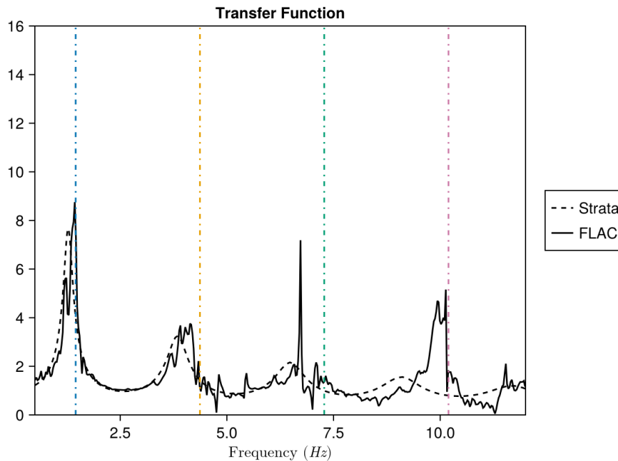
Σχήμα 3.7: Συνάρτηση Μεταφοράς Μη-Γραμμικής Ανάλυσης
