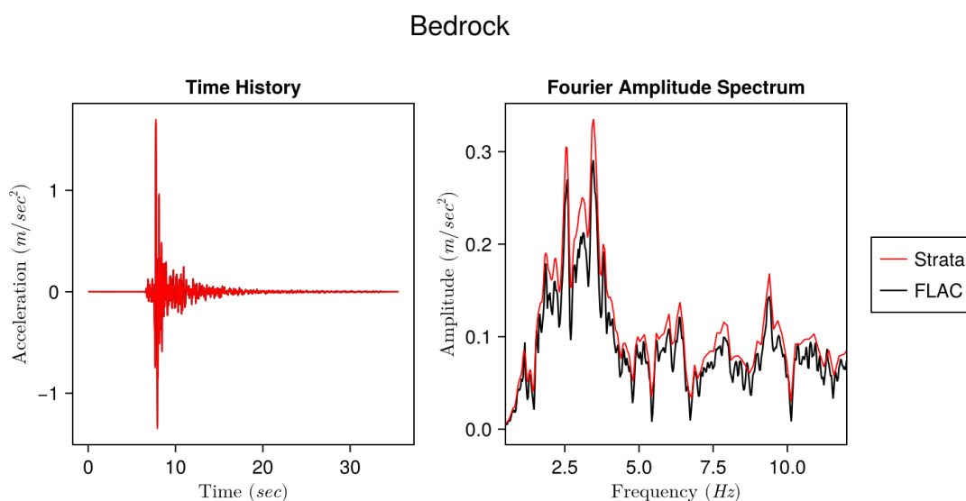
Σχήμα 3.3: Εισαγόμενη Χρονοϊστορία Βραχώδους Υποβάθρου
