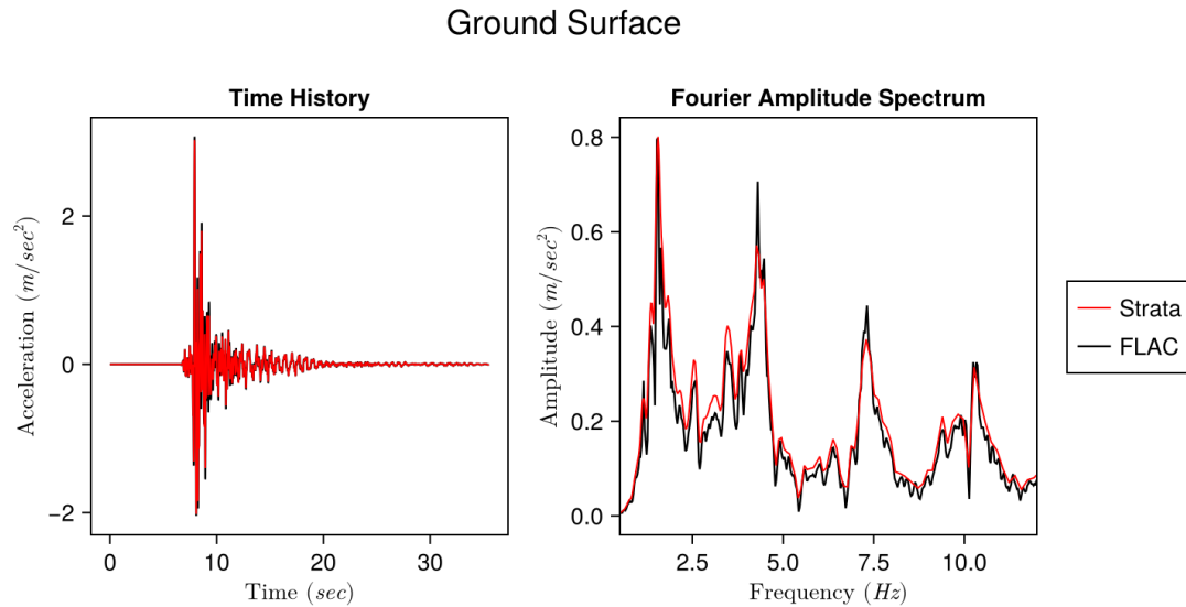
Σχήμα 3.4: Επιφανειακή Απόκριση Ελαστικής Ανάλυσης
