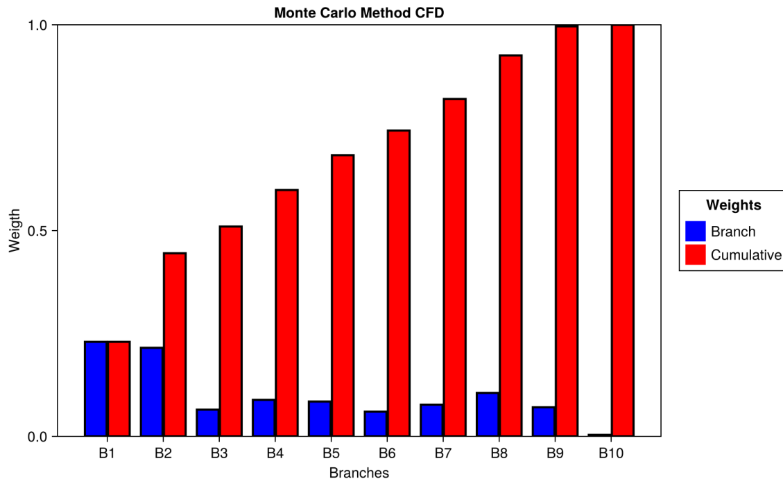
Σχήμα 2.8: Παράδειγμα της Μεθόδου Monte Carlo
