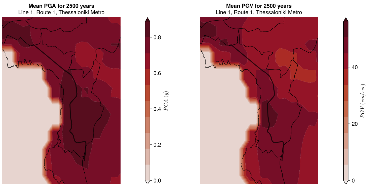
Σχήμα 2.15: Χάρτες Μέσων PGA-PGV V_{s30} ESRM20
