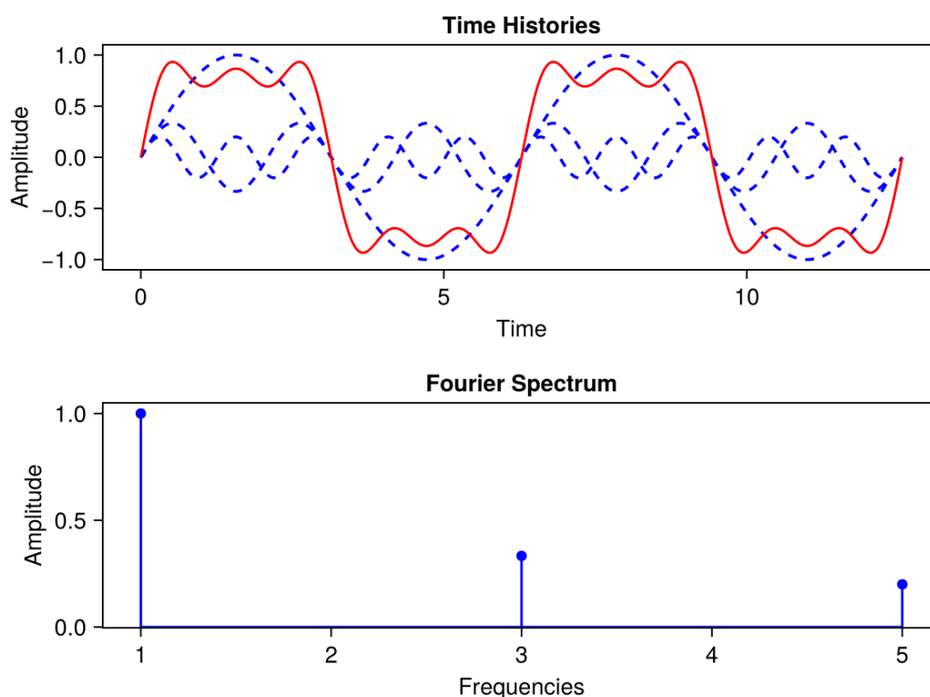
Σχήμα 3.2: Παράδειγμα Μετασχηματισμού Fourier
