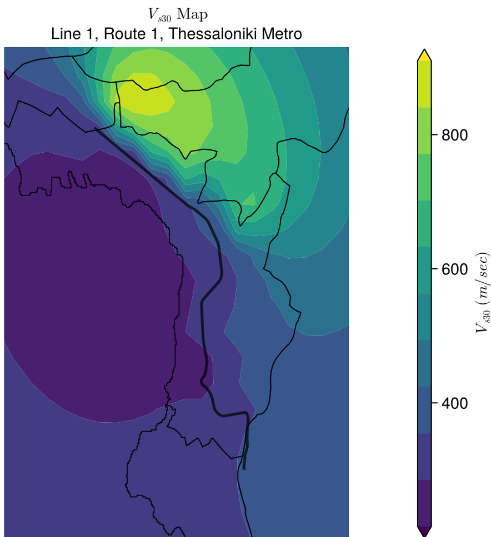
Σχήμα 2.5: Χάρτης τιμών V_{s30} (Τιμές Γεωτρήσεων)
