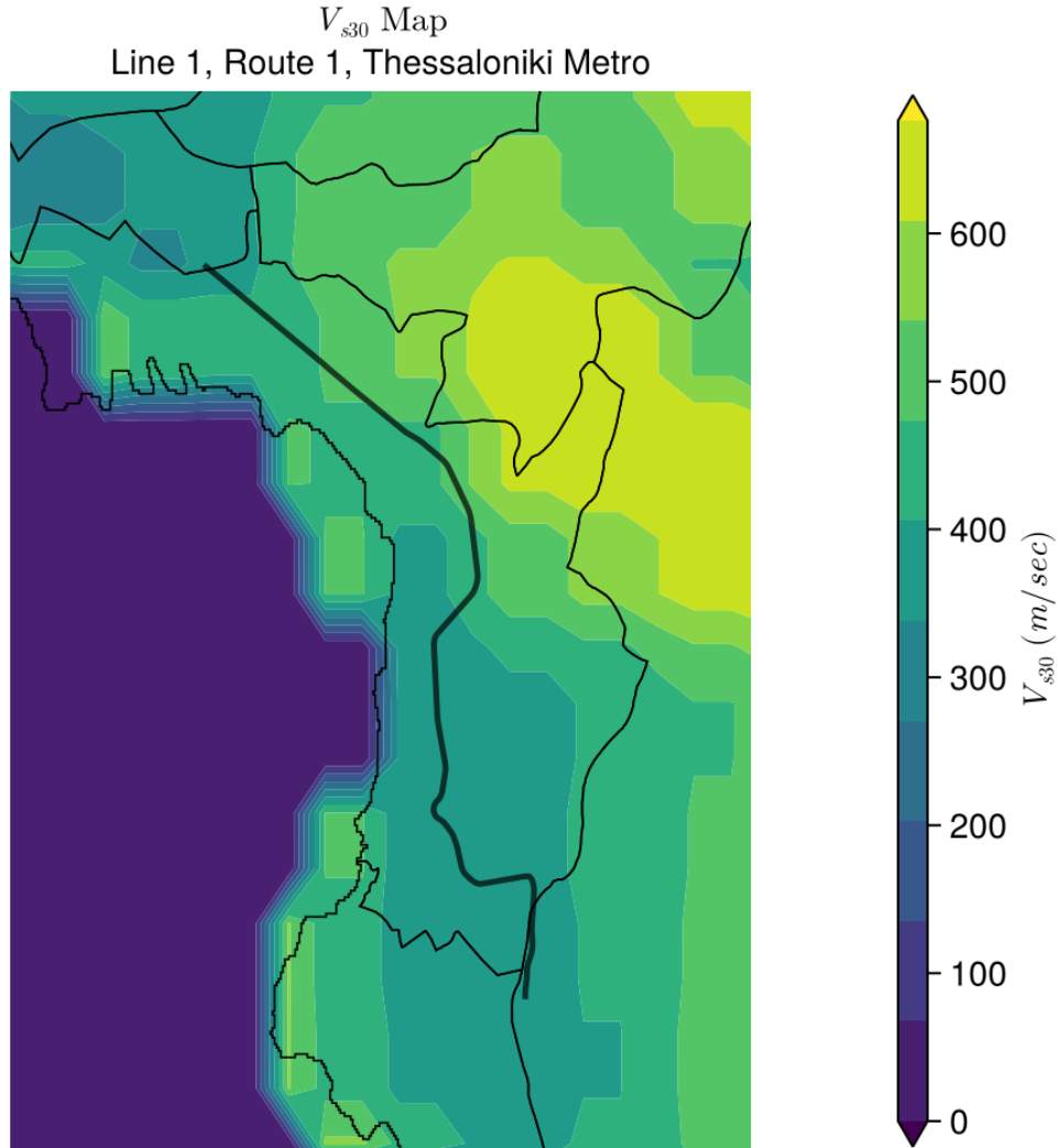
Σχήμα 2.6: Χάρτης τιμών V_{s30} (ESRM20 Sitemodel)
