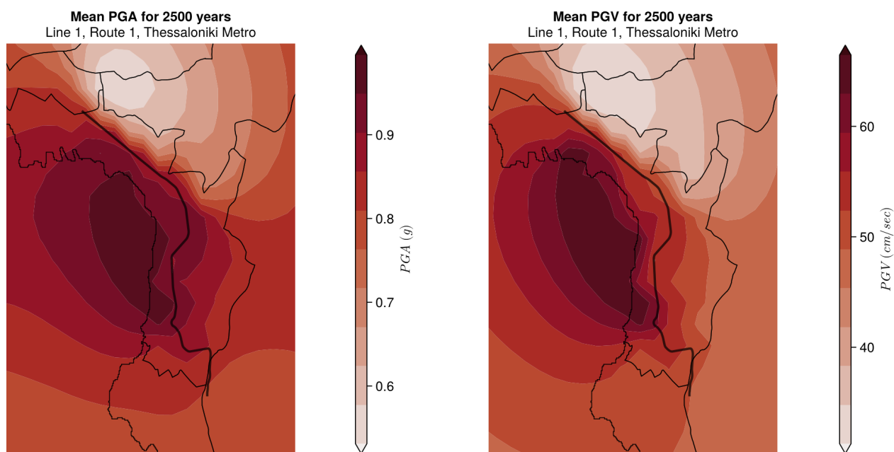
Σχήμα 2.14: Χάρτες Μέσων PGA-PGV Γεωτρήσεων
