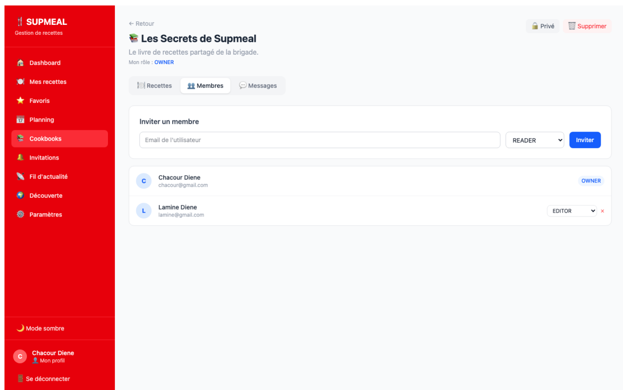
Gestion des membres d'un cookbook
