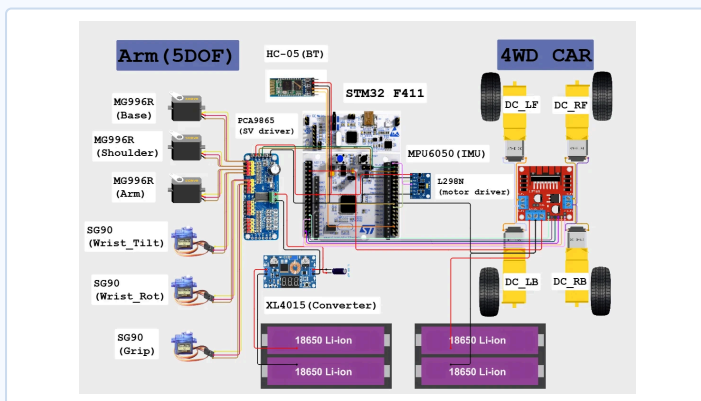
발표자료의 전체 배선도
