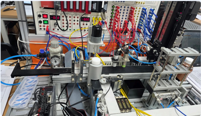
프로젝트에 사용한 PLC·모션·컨베이어 장비
