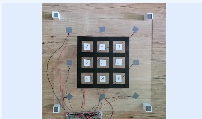
400×400mm 아크릴판 · 직접 구성한 실험 장치
