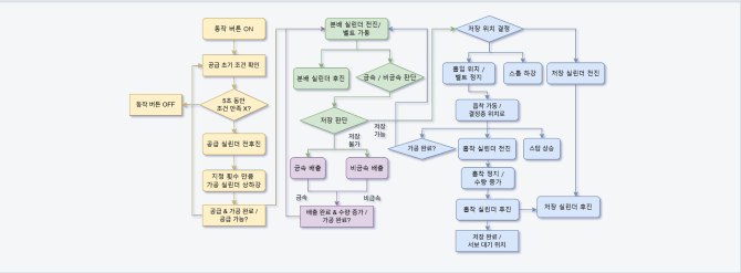
저장 판단과 적재 동작의 병렬 시퀀스
