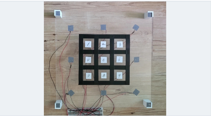
400×400mm 아크릴판 · 직접 구성한 실험 장치
