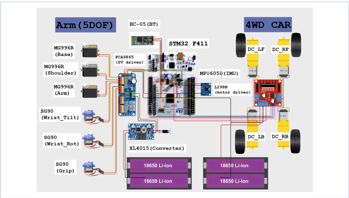
로봇팔·이동체의 전체 배선도
