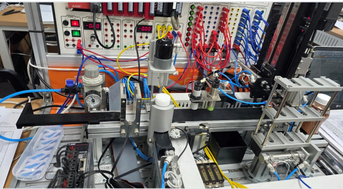
프로젝트에 사용한 PLC · 모션 · 컨베이어 장비
