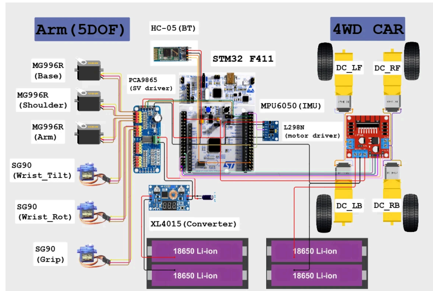
로봇팔·이동체의 전체 배선도
