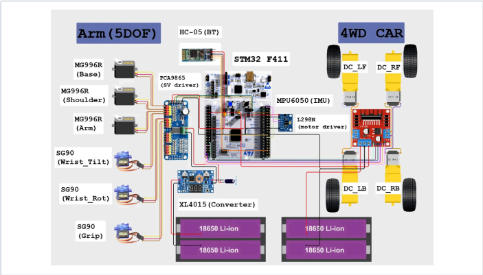
그림 2. 로봇팔·이동체의 전체 배선도
