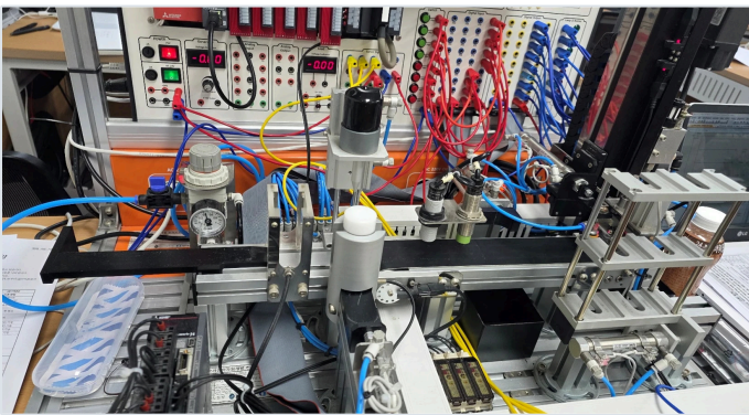
그림 6. 프로젝트에 사용한 PLC·모션·컨베이어 장비
