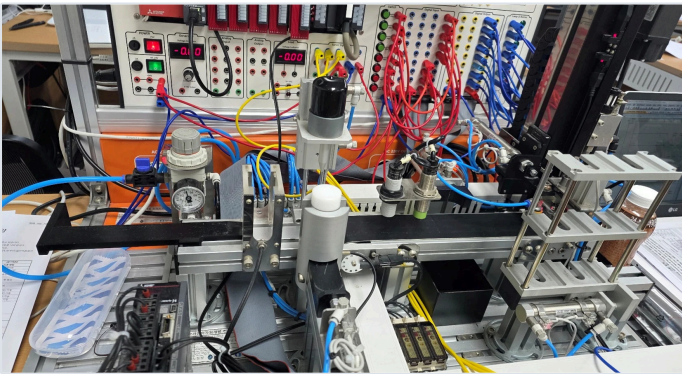
프로젝트에 사용한 PLC·모션·컨베이어 장비
