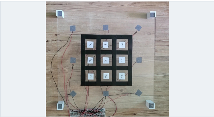
400×400mm 아크릴판 · 직접 구성한 실험 장치
