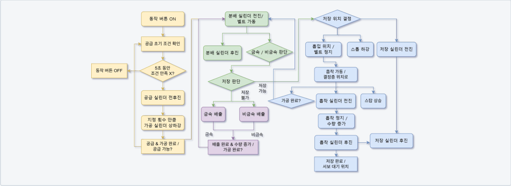
그림 7. 저장 판단과 적재 동작의 병렬 시퀀스
