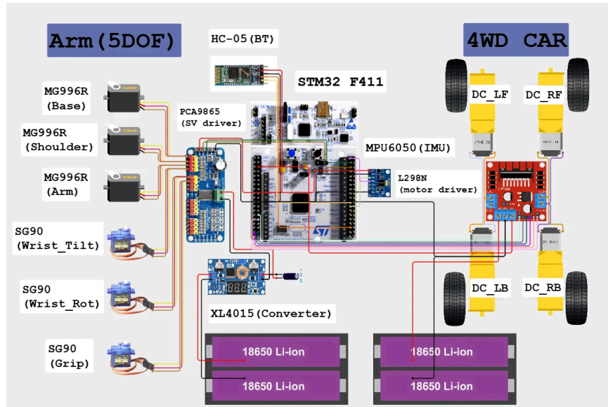
그림 2. 로봇팔·이동체의 전체 배선도
