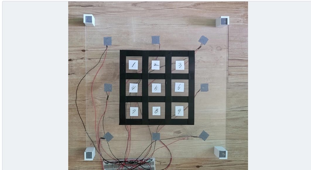
그림 10. 400×400mm 아크릴판 · 직접 구성한 실험 장치
