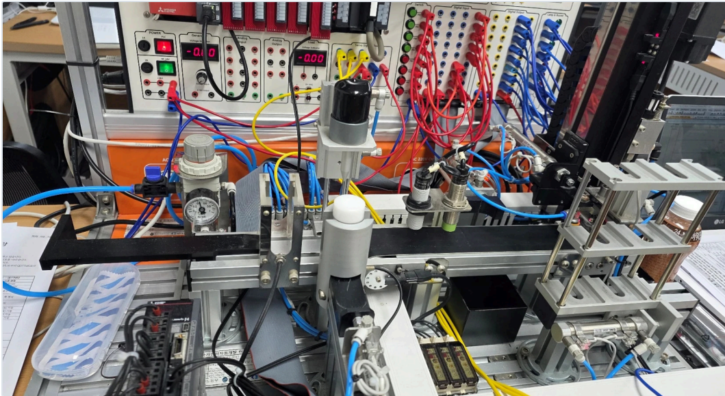
그림 6. 프로젝트에 사용한 PLC·모션·컨베이어 장비
