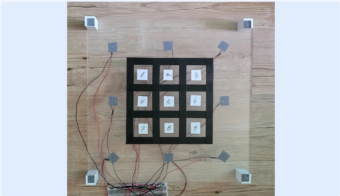
400×400mm 아크릴판 · 직접 구성한 실험 장치
