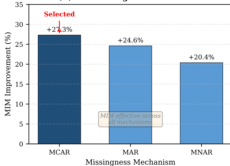
(D) L4: Missingness Mechanism
