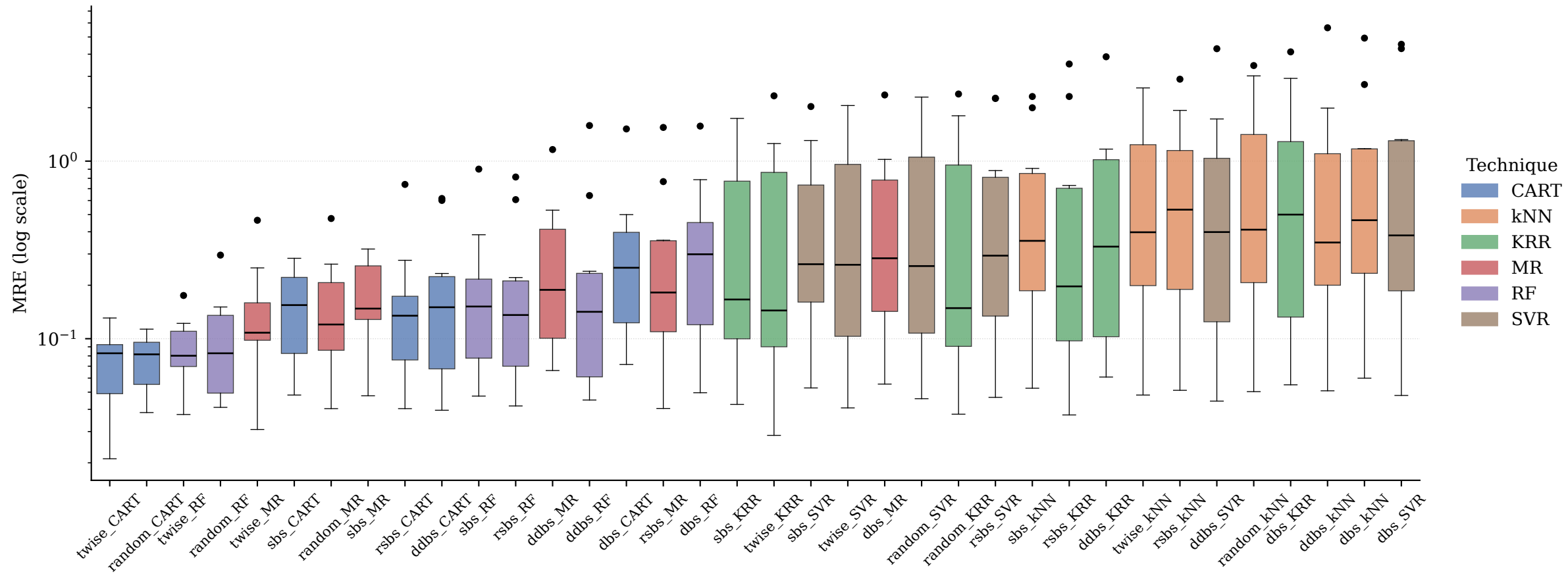
MRE - t = 3
