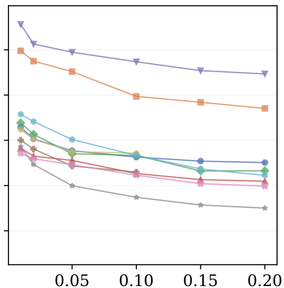
SVR
