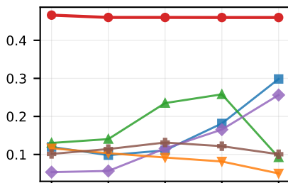
Benzene
