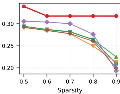
SPMotif-0.9
