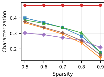
SPMotif-0.7
