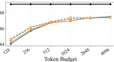
(d) LongBench, Qwen2.5-7b-instruct
