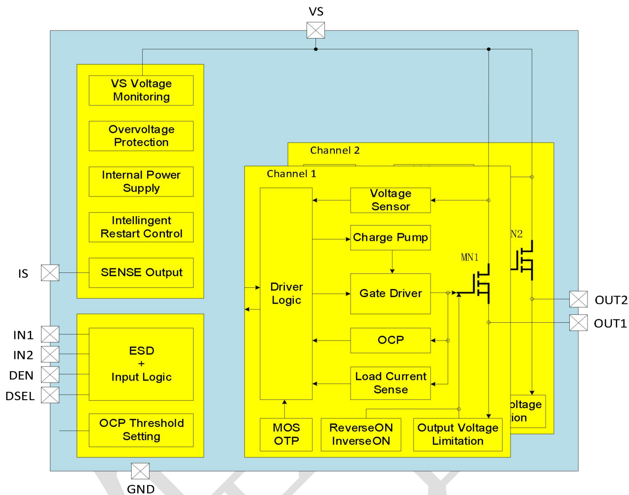
图 3 功能框图
