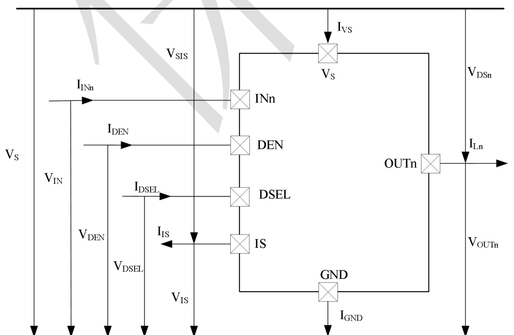
图 3 功能框图
