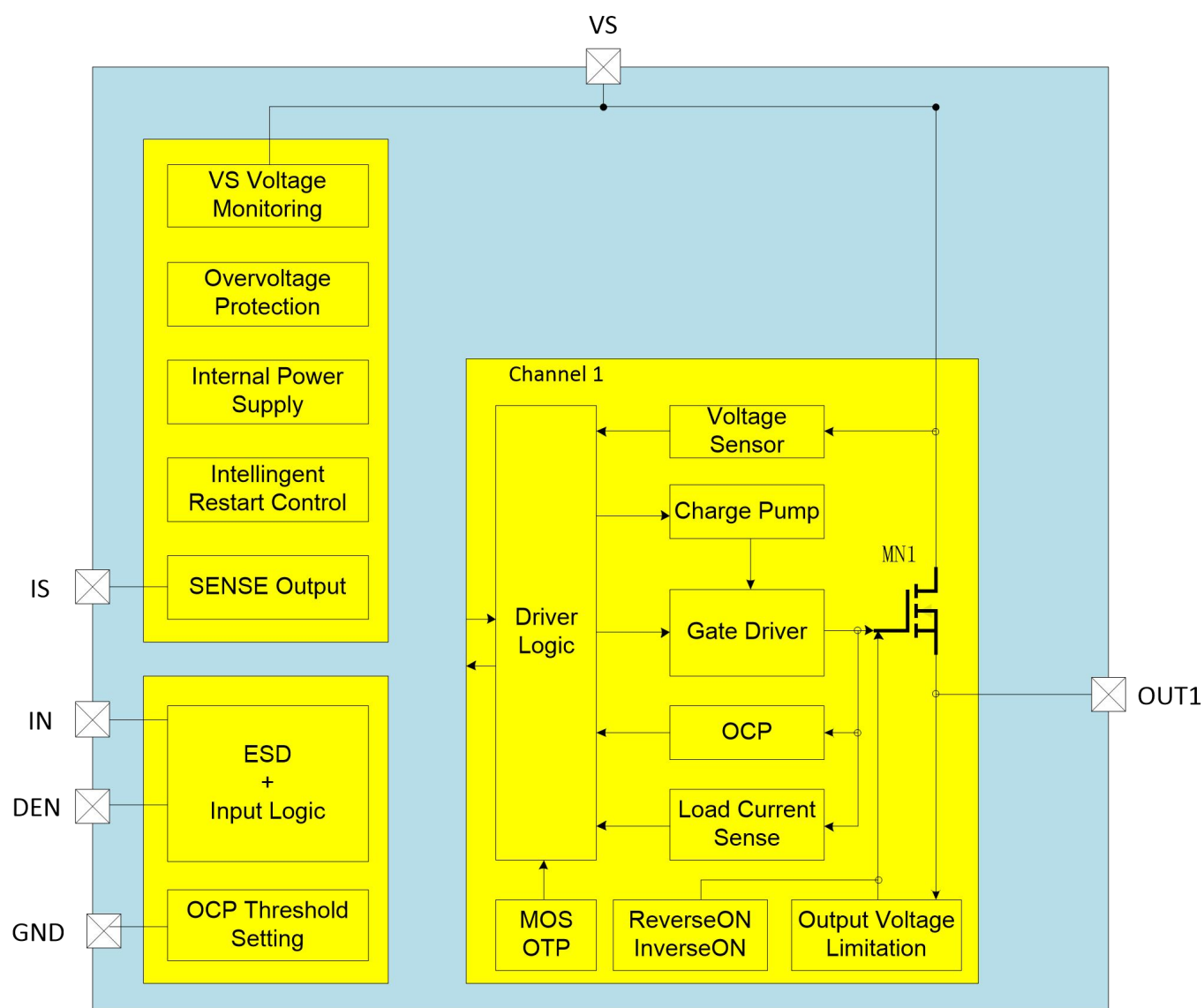
图 3 功能框图
