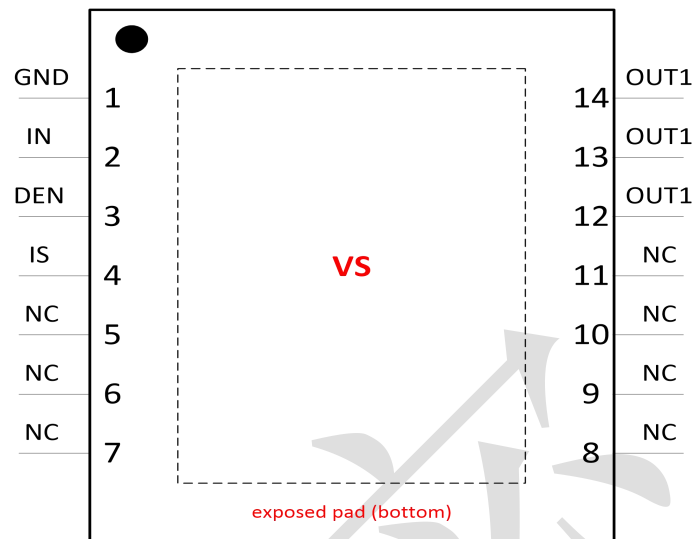
图 2 引脚配置
