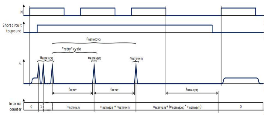
图 7 过功率重启策略时序-通道输入为 PWM 信号
