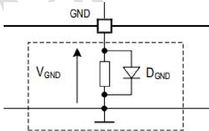
图 10 防电池反接二极管和电阻示意图
