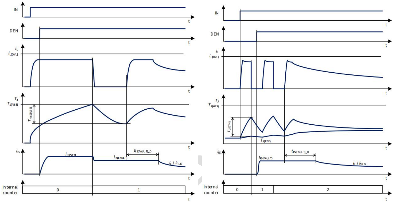
图 9 绝对过温保护(左)和动态过温保护(右)
