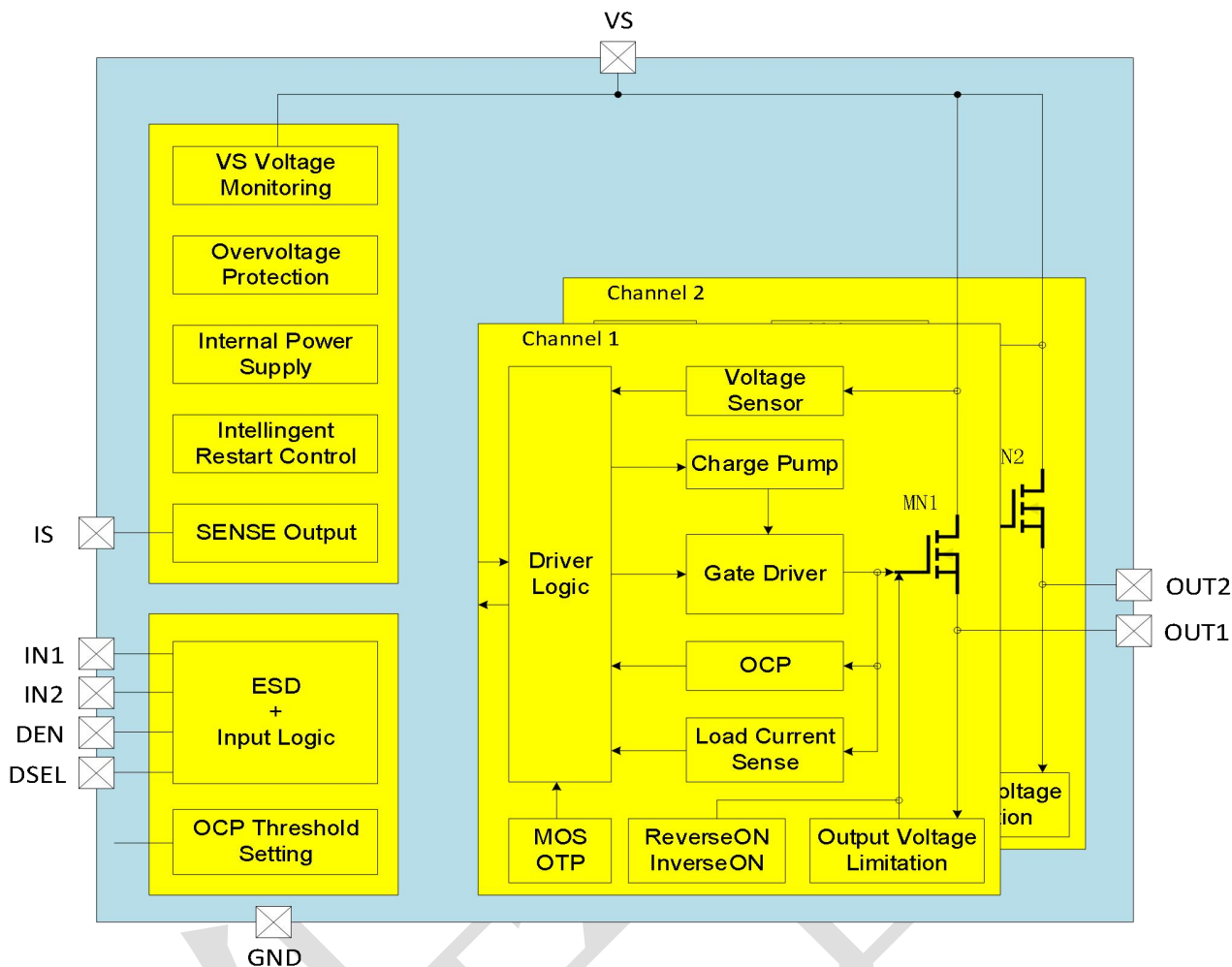
图 3 功能框图
