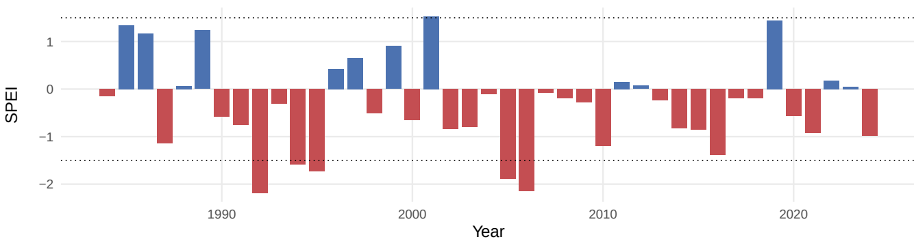
(d) SPEI-12, October
