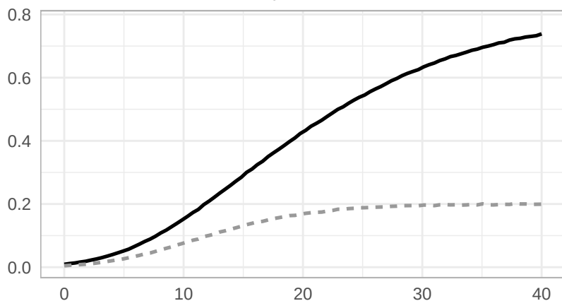
F 7 Gumbel
