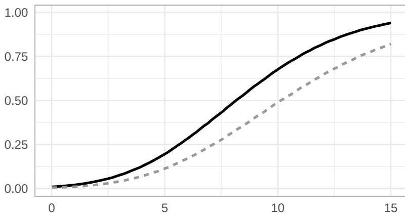
F 7 Gumbel
