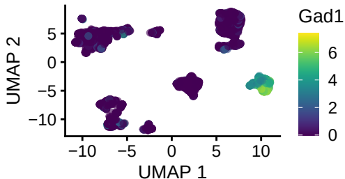
cluster 1 – Gad1
