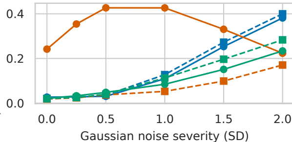
Digits
