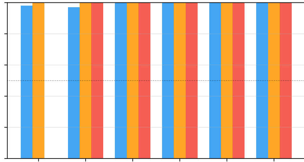
kmerseek k26
