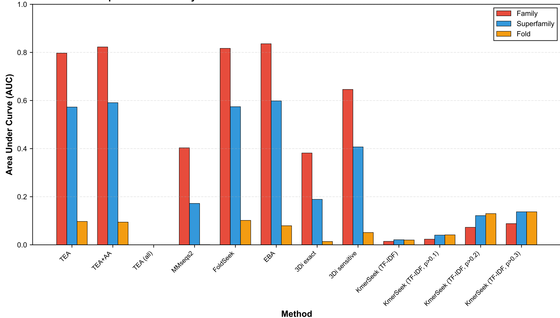
Benchmark Comparison: Sensitivity AUC
