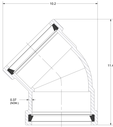
6" 45 Bend GxG
