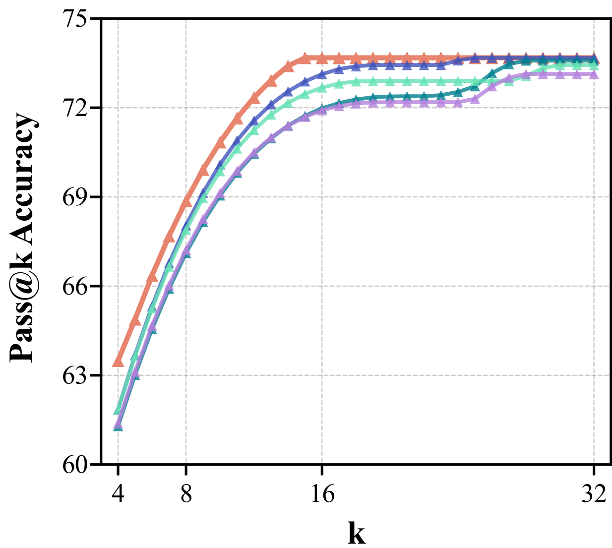
MathVista
