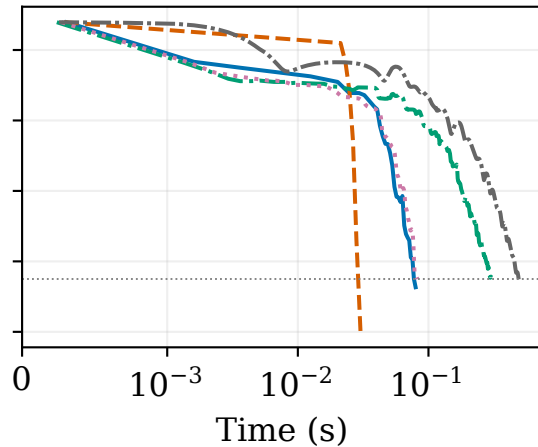
(b) WDBC
