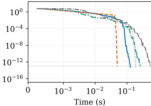
(a) C0
