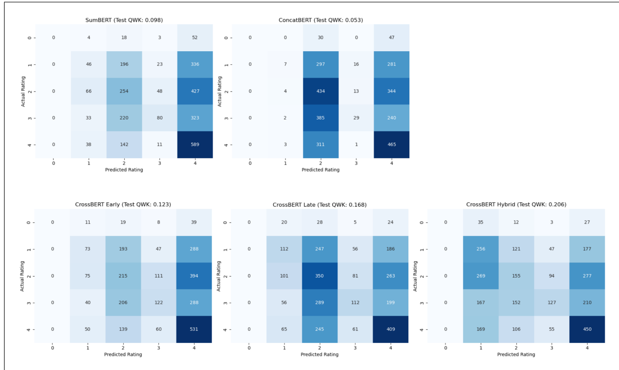
Abb. 9: Konfusionsmatrizen der Modelle auf dem Petfinder-Testdatensatz. Die Titel zeigen den jeweiligen Test-QWK.
