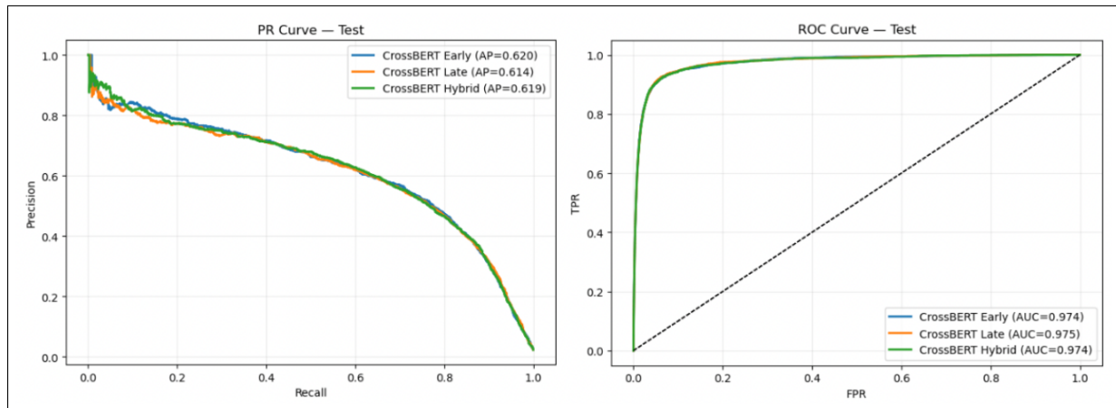
Abb. 7: Vergleich der Metrik-Verläufe für CrossBERT Early, Late und Hybrid.
