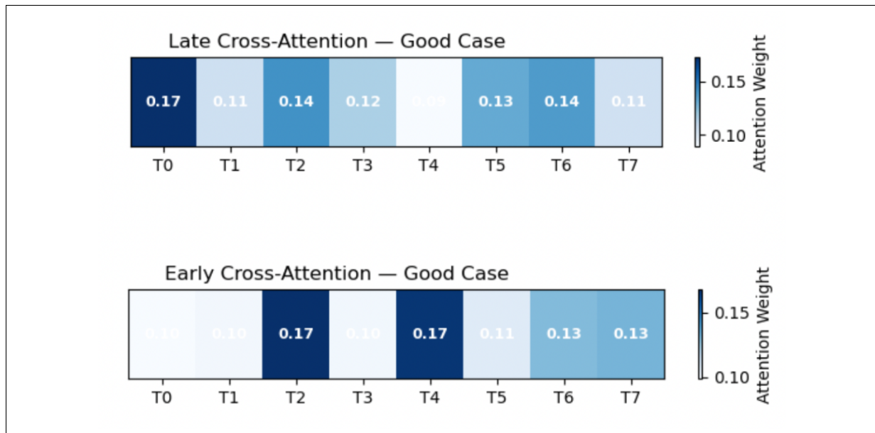
Abb. 8: Attention-Weights im Good Case.
