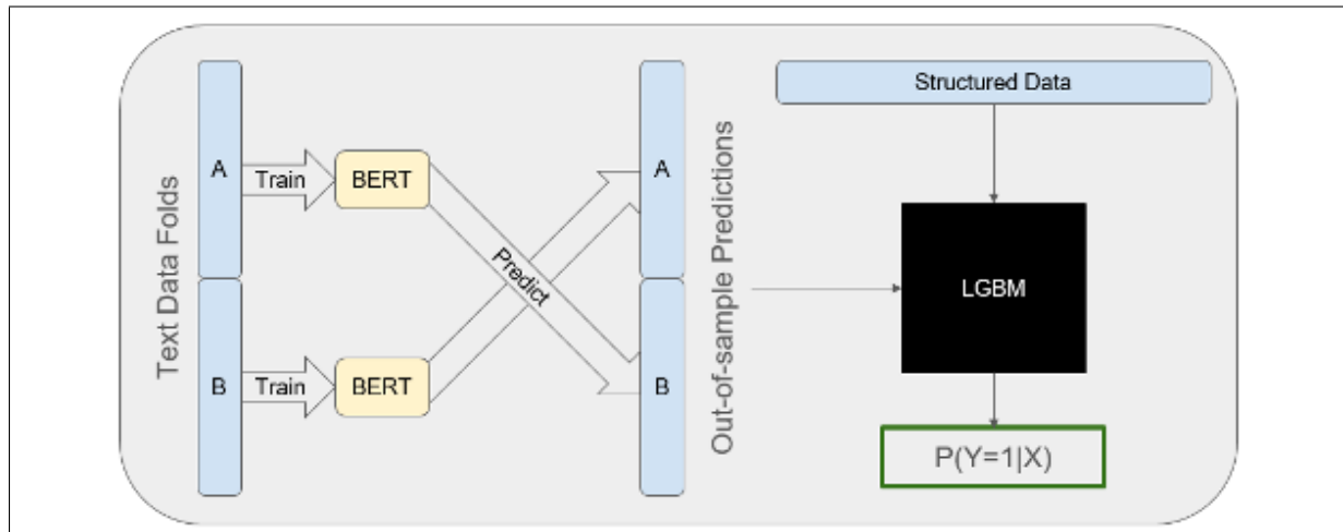
Abb. 12: Schematische Darstellung der CrossFitter-Modellarchitektur im produktiven Einsatz. Quelle: [Fue24].
